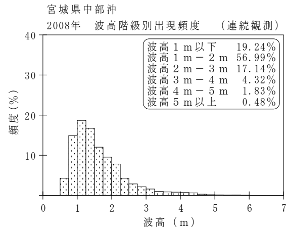
付図-B.1.63 宮城県中部沖 波候特性図 (連続観測)
