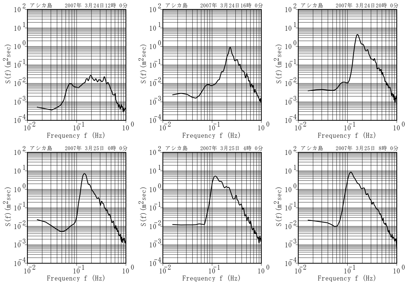
付図-A. 5. 43 アシカ島 代表的な高波期間中のスペクトル
