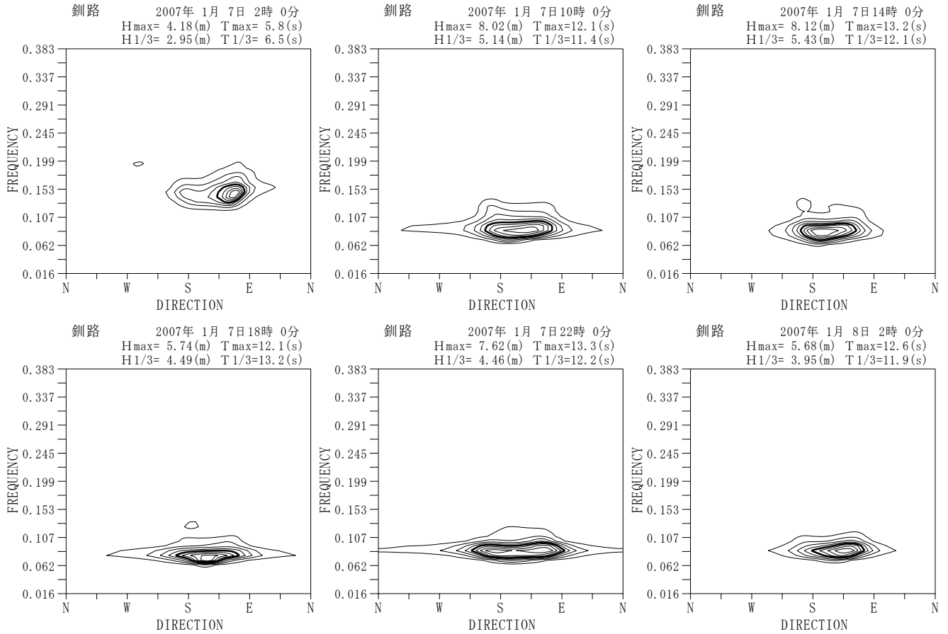
付図-A.5.28 鉧路 代表的な高波期間中の方向スペクトル
