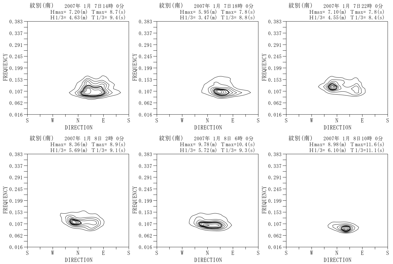
付図-A.5.27 紋別(南) 代表的な高波期間中の方向スペクトル
