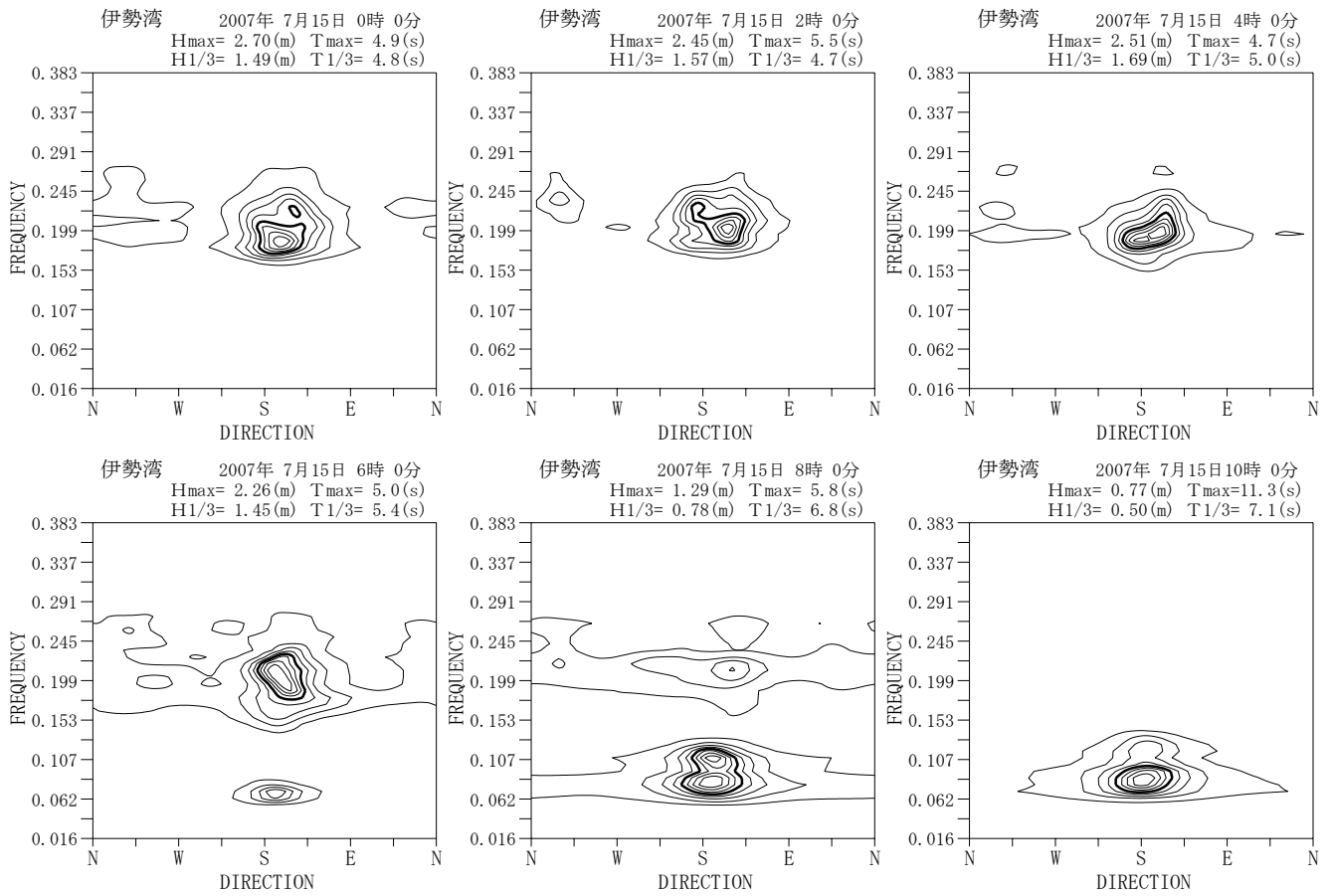
付図-A. 5. 48 伊勢湾 代表的な高波期間中の方向スペクトル
