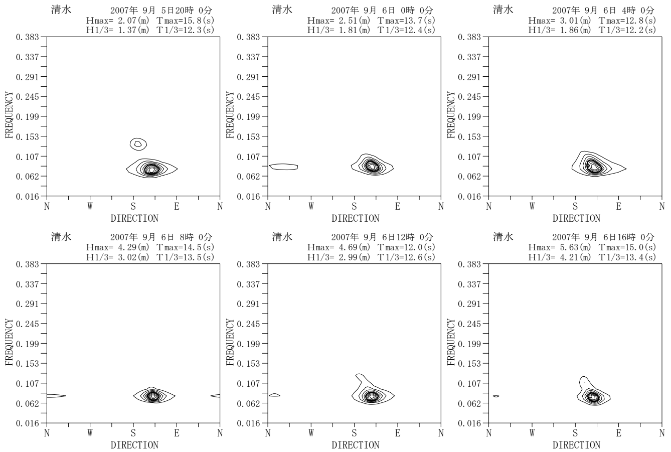
付図—A. 5. 46 清水 代表的な高波期間中の方向スペクトル
