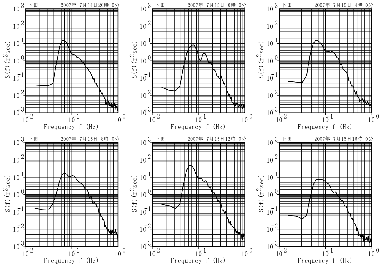
付図-A.5.45 下田 代表的な高波期間中のスペクトル
