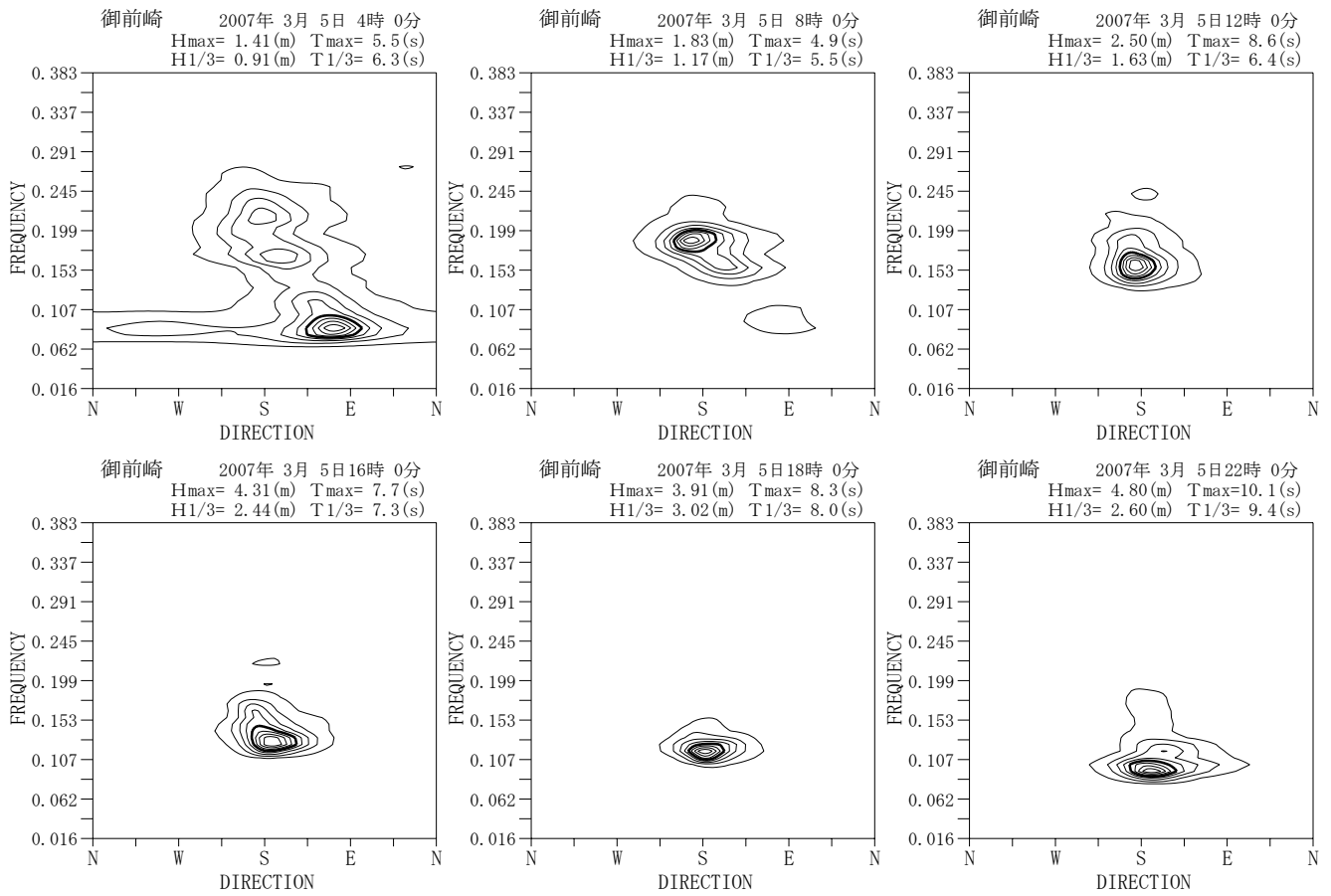
付図-A. 5. 47 御前崎 代表的な高波期間中の方向スペクトル
