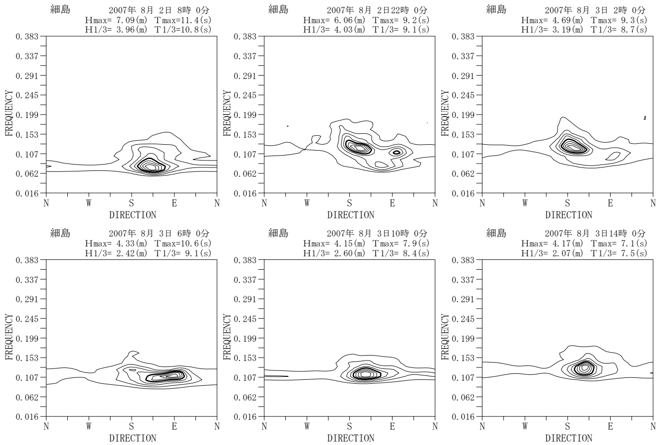
付図—A. 5.56 細島 代表的な高波期間中の方向スペクトル
