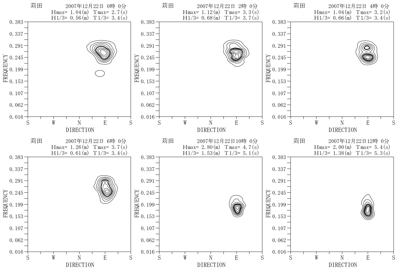
付図-A. 5.55 菊田 代表的な高波期間中の方向スペクトル
