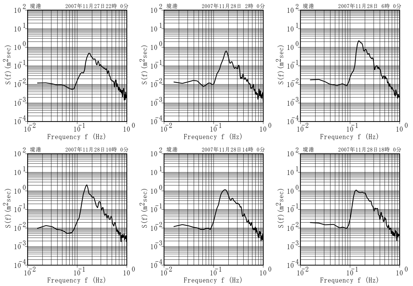
付図-A.5.19 境港 代表的な高波期間中のスペクトル
