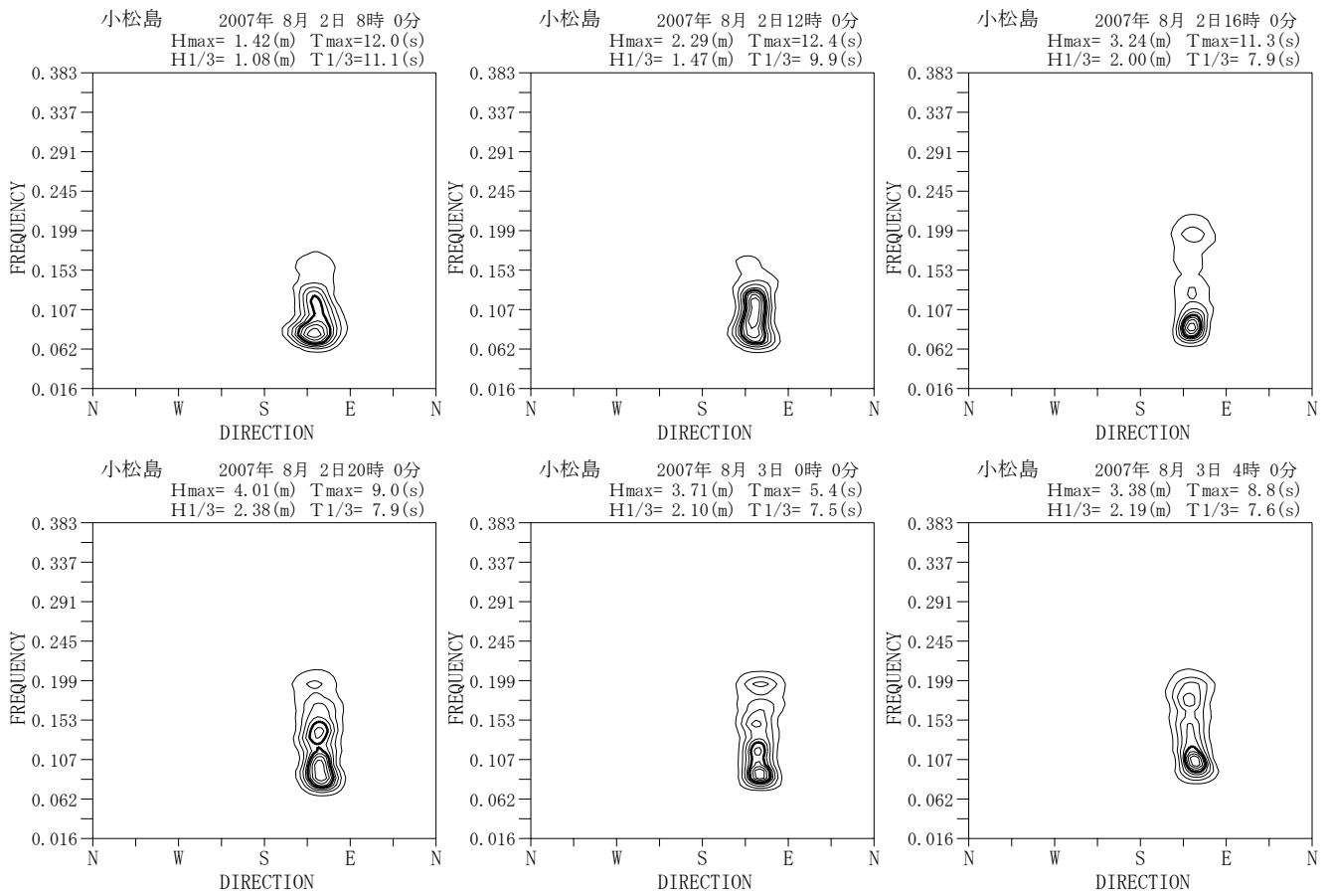
付図-A. 5. 51 小松島 代表的な高波期間中の方向スペクトル
