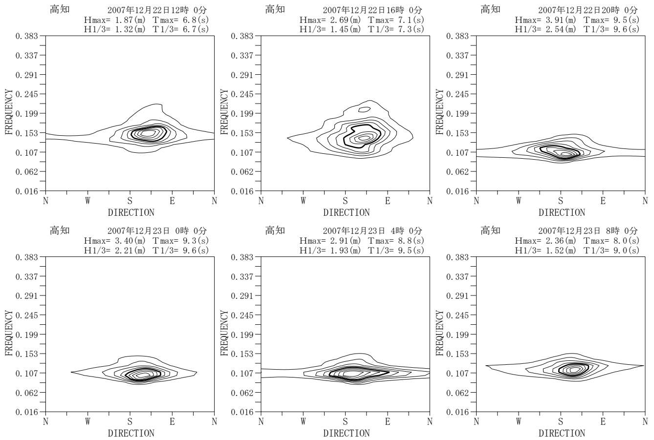
付図-A. 5.53 高知 代表的な高波期間中の方向スペクトル
