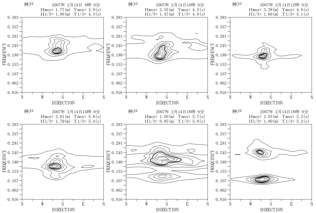
付図-A. 5.50 神戸 代表的な高波期間中の方向スペクトル
