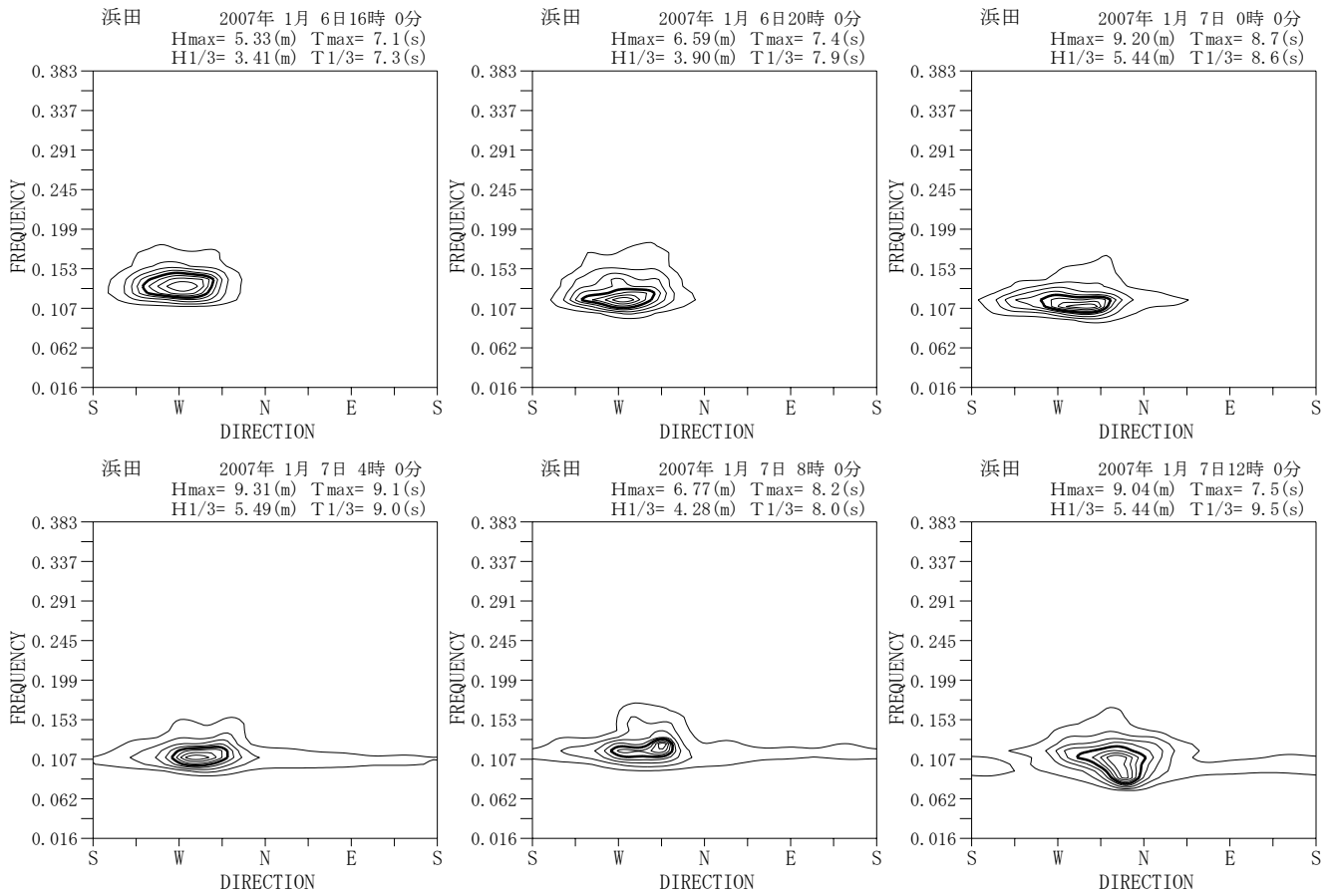
付図-A. 5. 20 浜田 代表的な高波期間中の方向スペクトル
