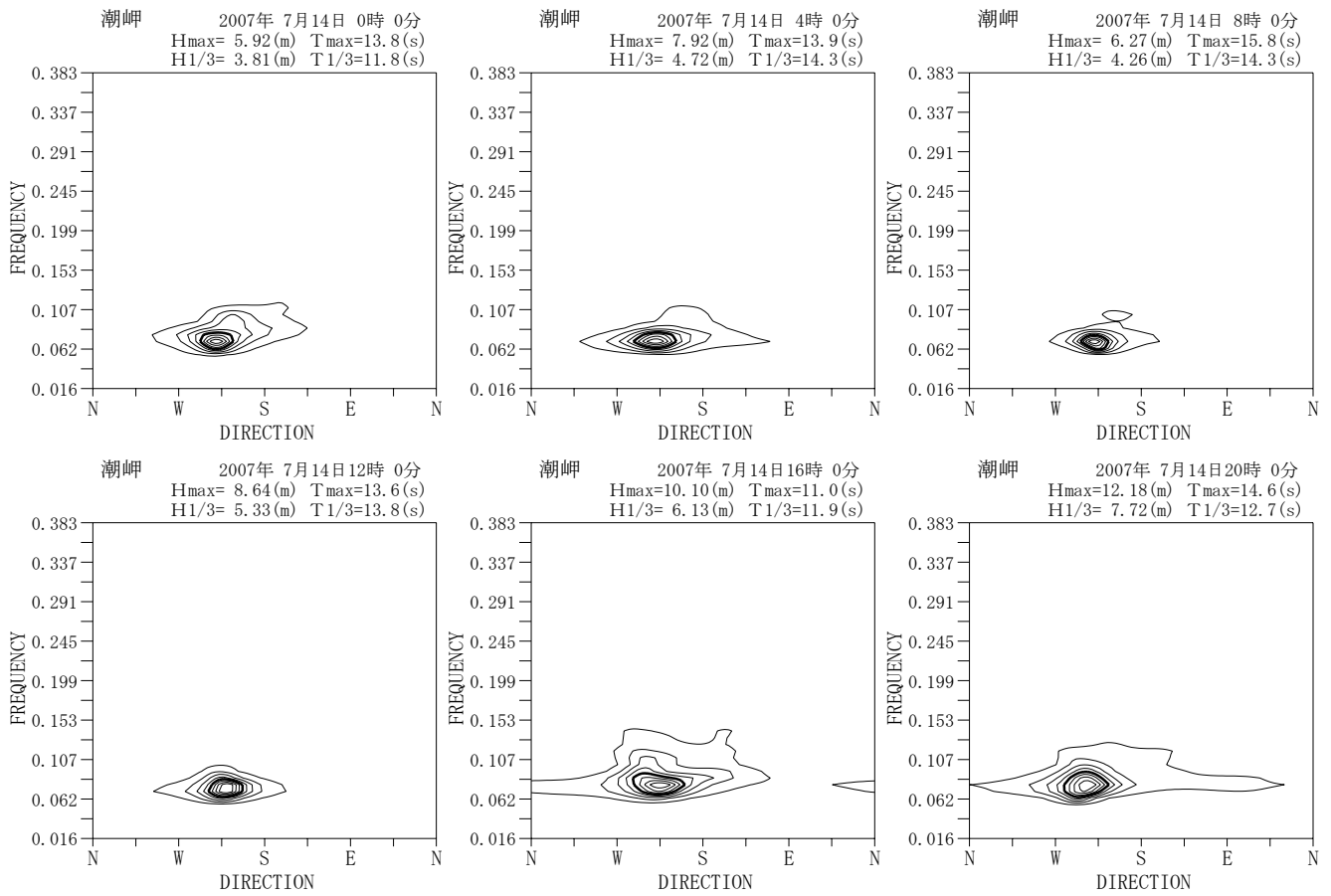
付図—A. 5. 49 潮岬 代表的な高波期間中の方向スペクトル
