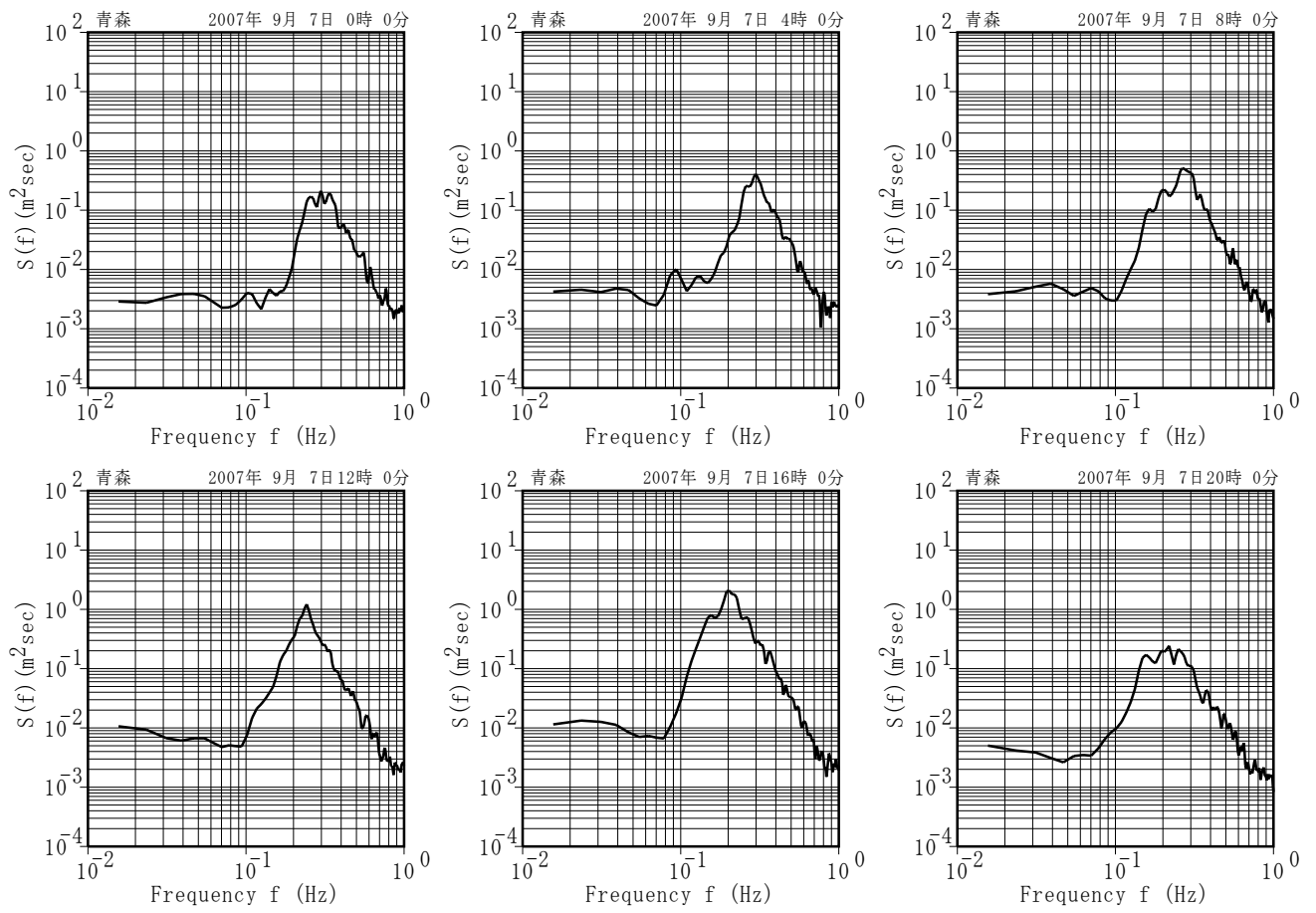
付図-A. 5. 4 青森 代表的な高波期間中のスペクトル
