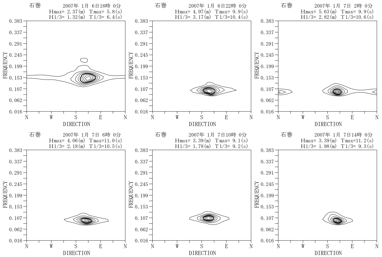
付図-A. 5.36 石巻 代表的な高波期間中の方向スペクトル
