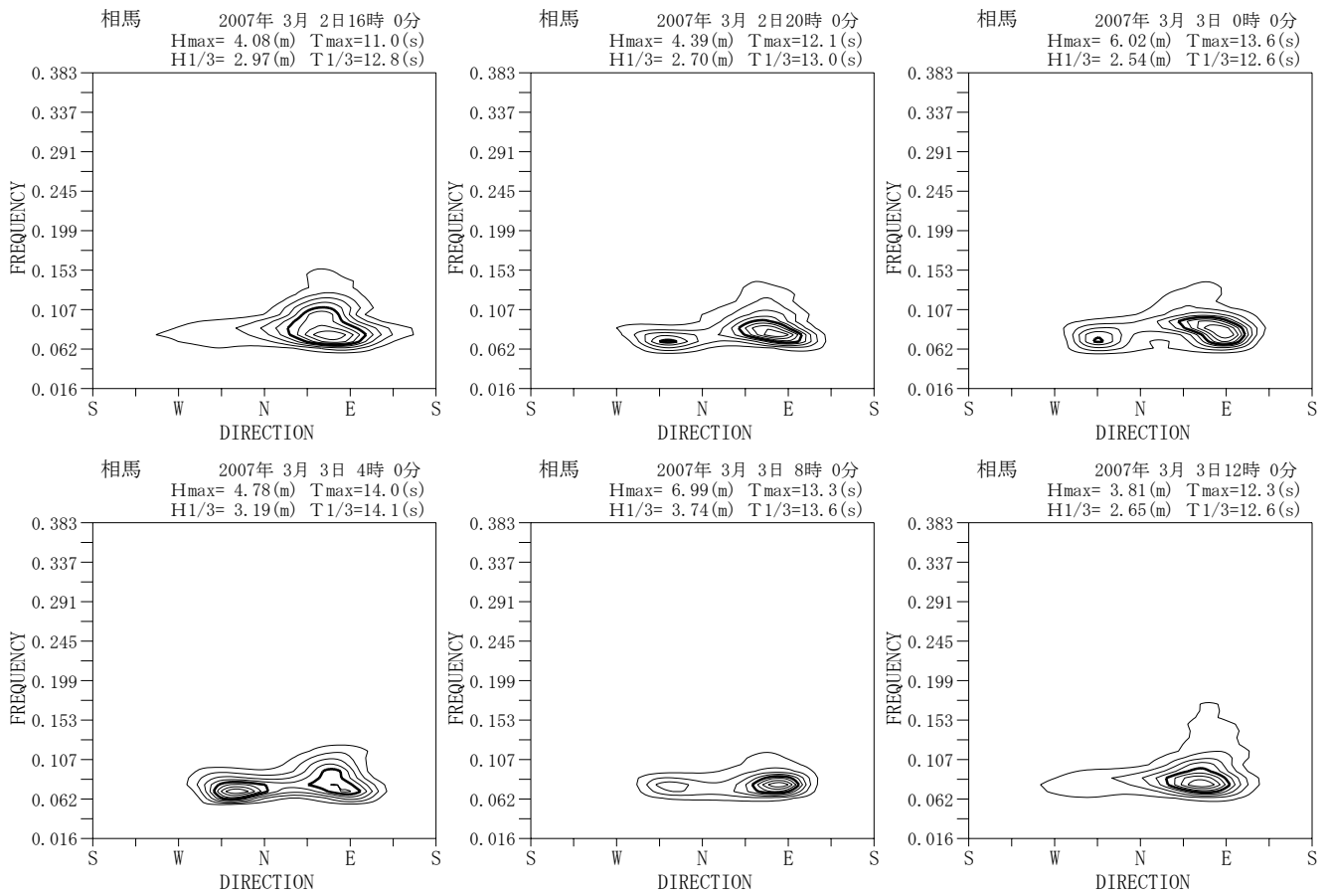
付図—A. 5. 38 相馬 代表的な高波期間中の方向スペクトル
