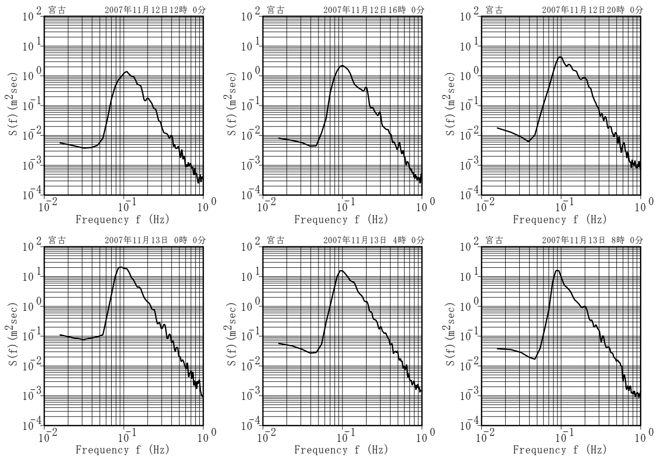
付図-A.5.34 宮古 代表的な高波期間中のスペクトル
