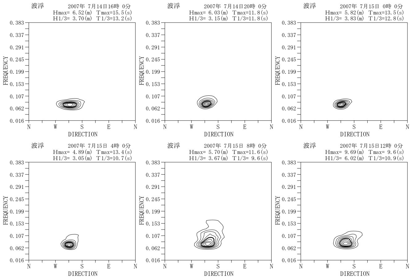
付図—A. 5.44 波浮 代表的な高波期間中の方向スペクトル
