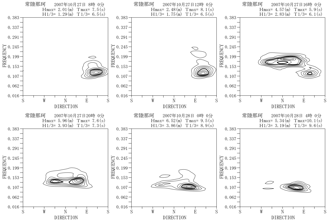
付図-A. 5. 40 常陸那珂 代表的な高波期間中の方向スペクトル
