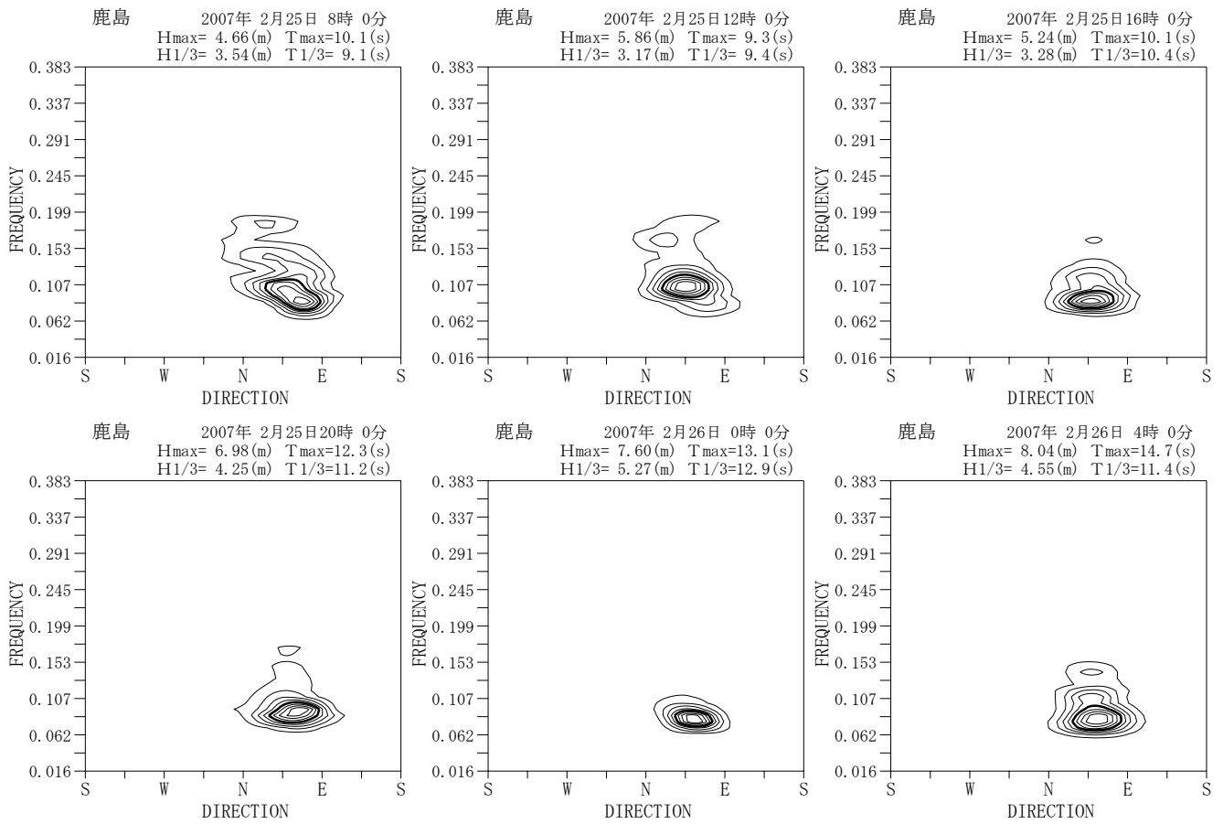
付図-A. 5. 41 鹿島 代表的な高波期間中の方向スペクトル
