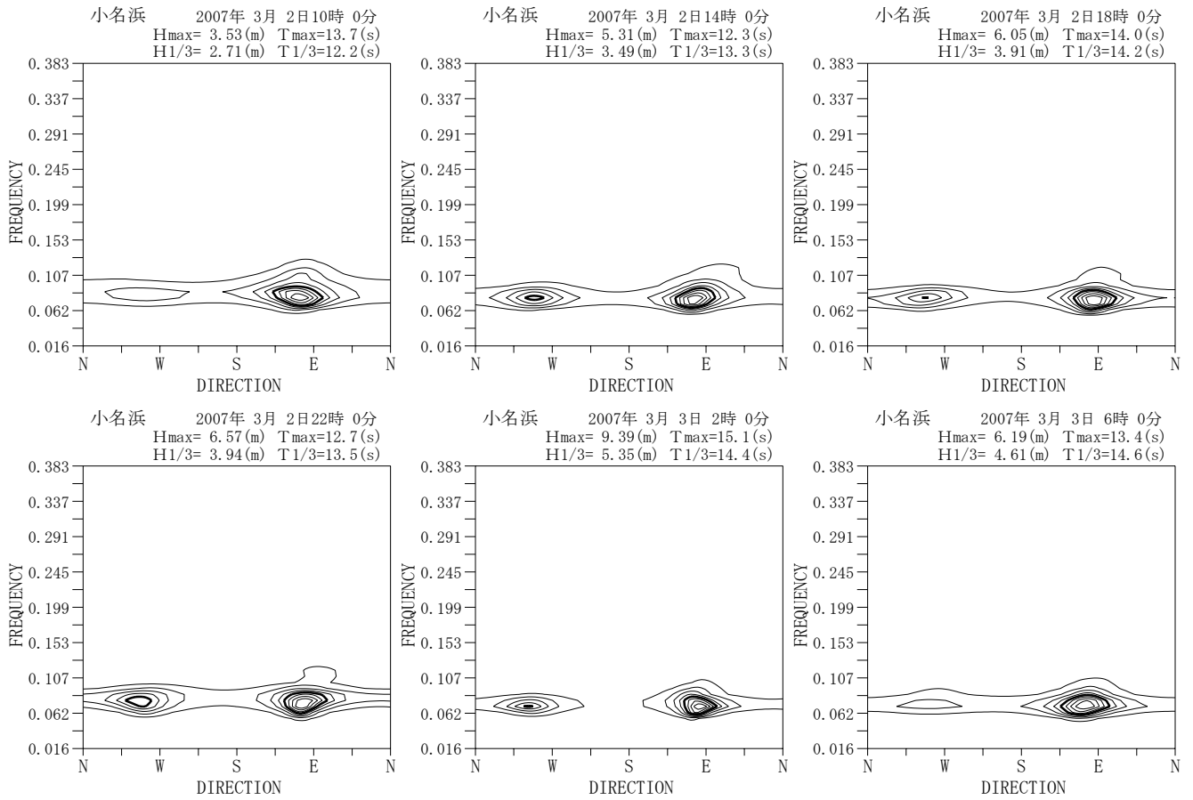
付図—A. 5. 39 小名浜 代表的な高波期間中の方向スペクトル
