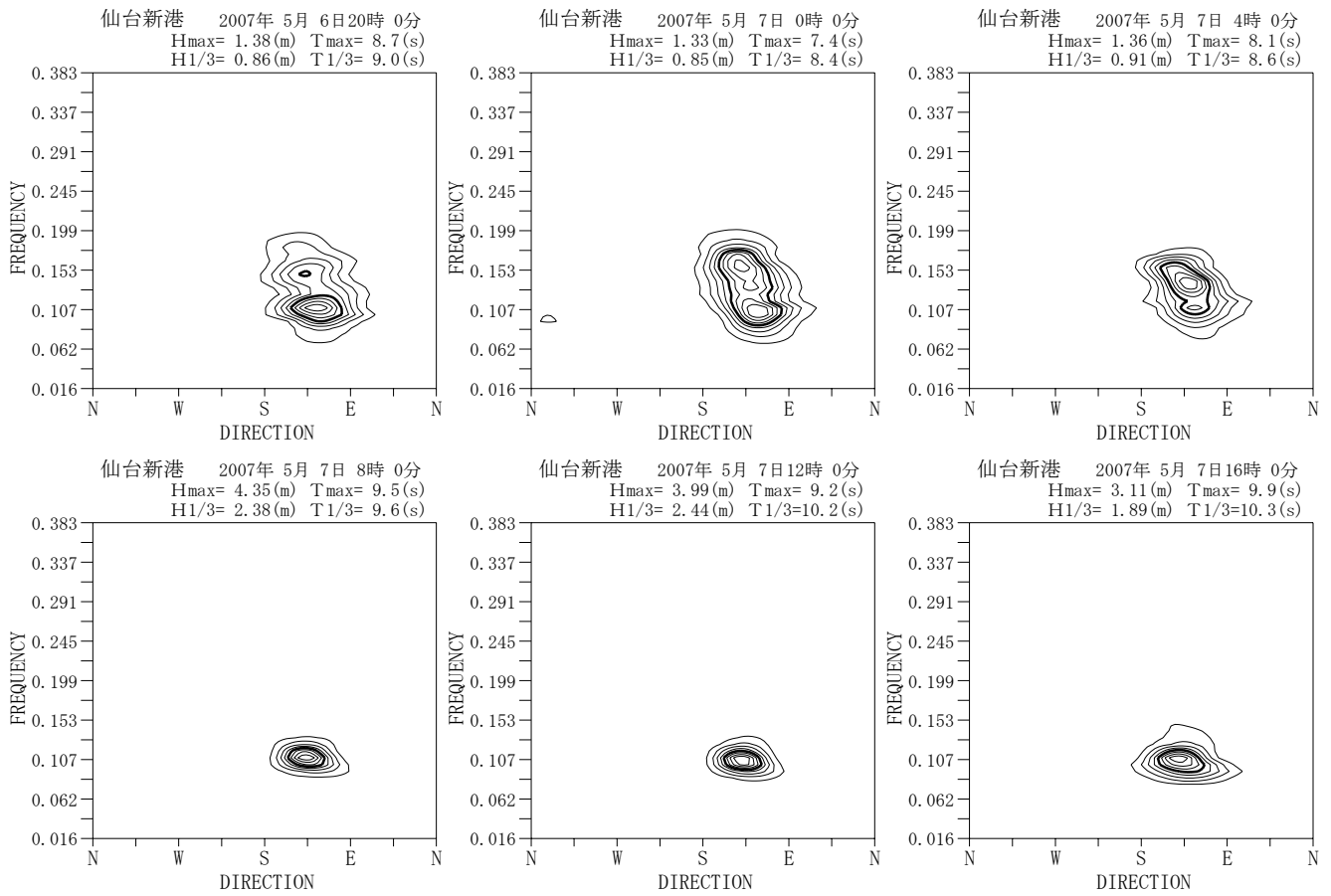
付図-A. 5. 37 仙台新港 代表的な高波期間中の方向スペクトル
