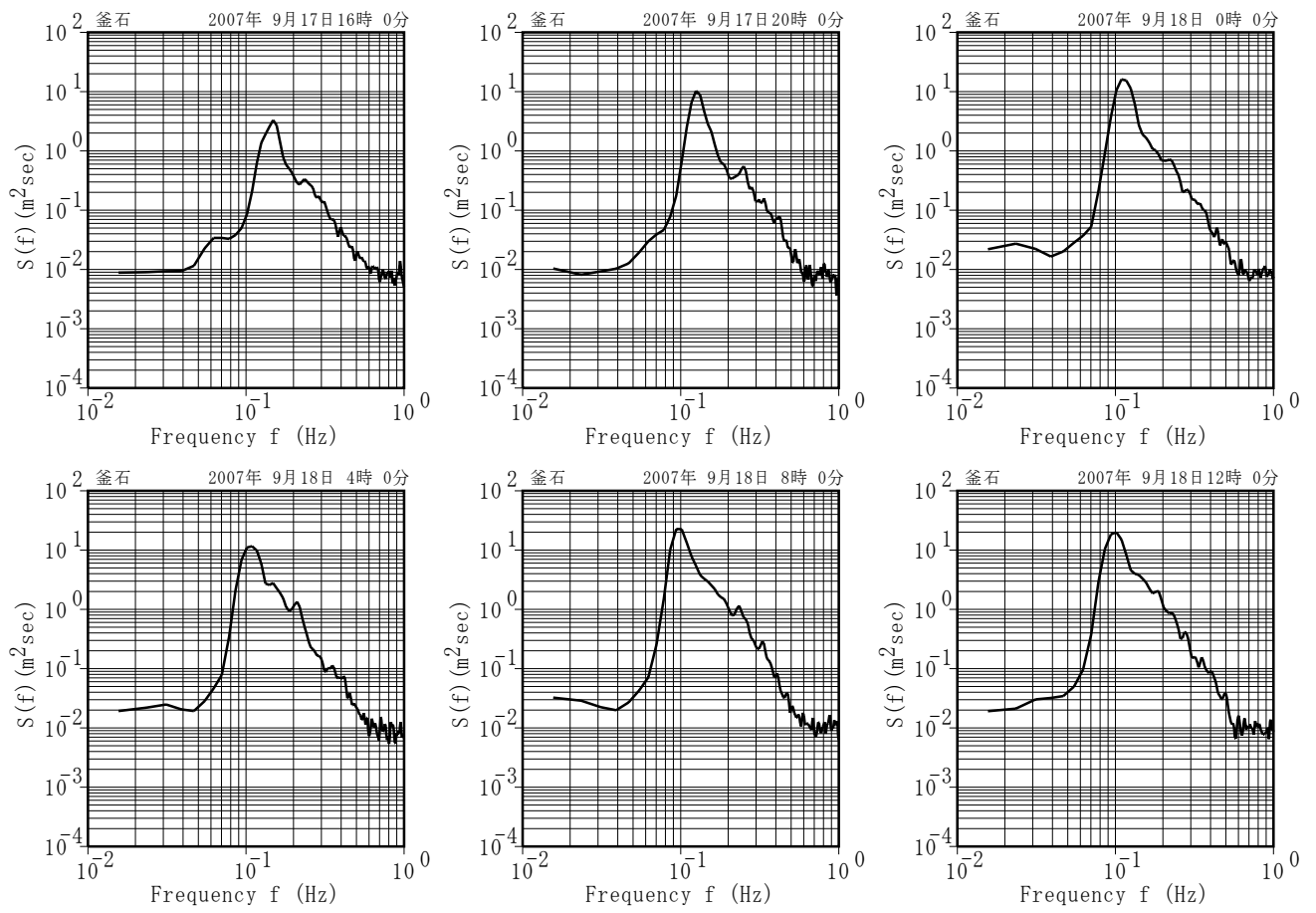
付図-A.5.35 釜石 代表的な高波期間中のスペクトル
