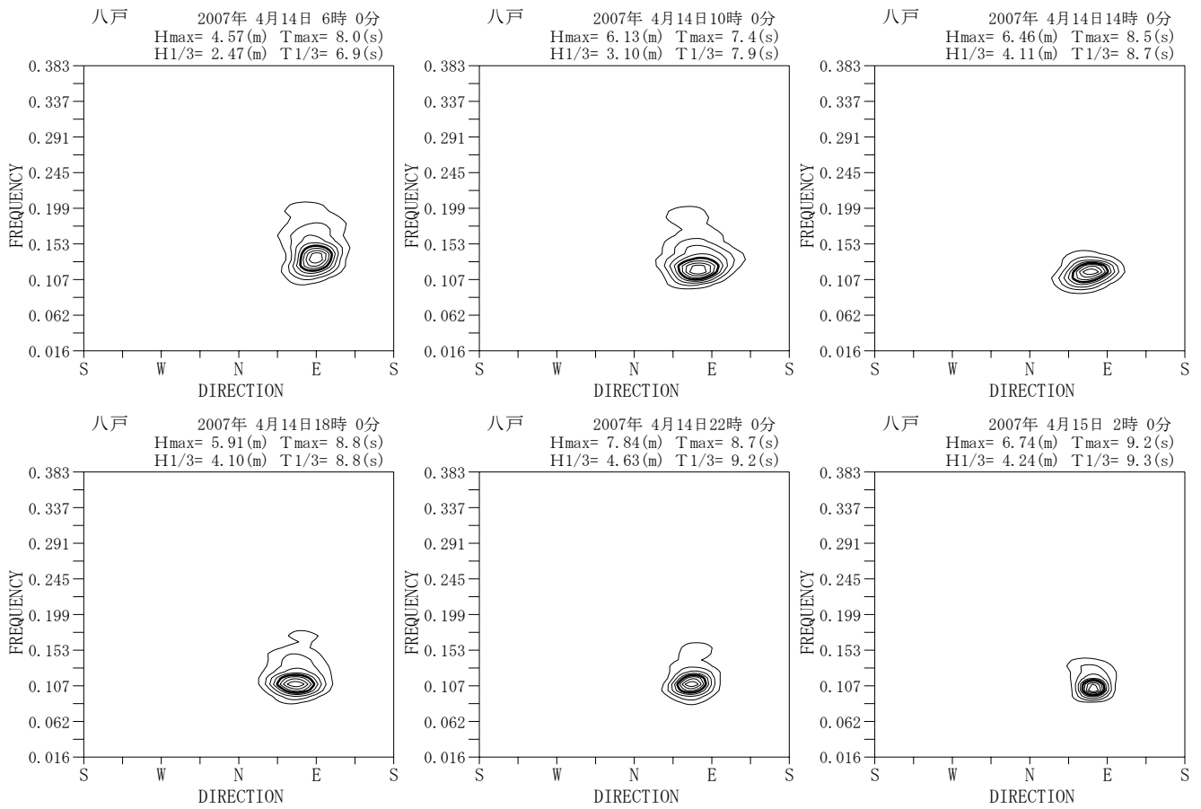
付図-A. 5. 32 八戸 代表的な高波期間中の方向スペクトル
