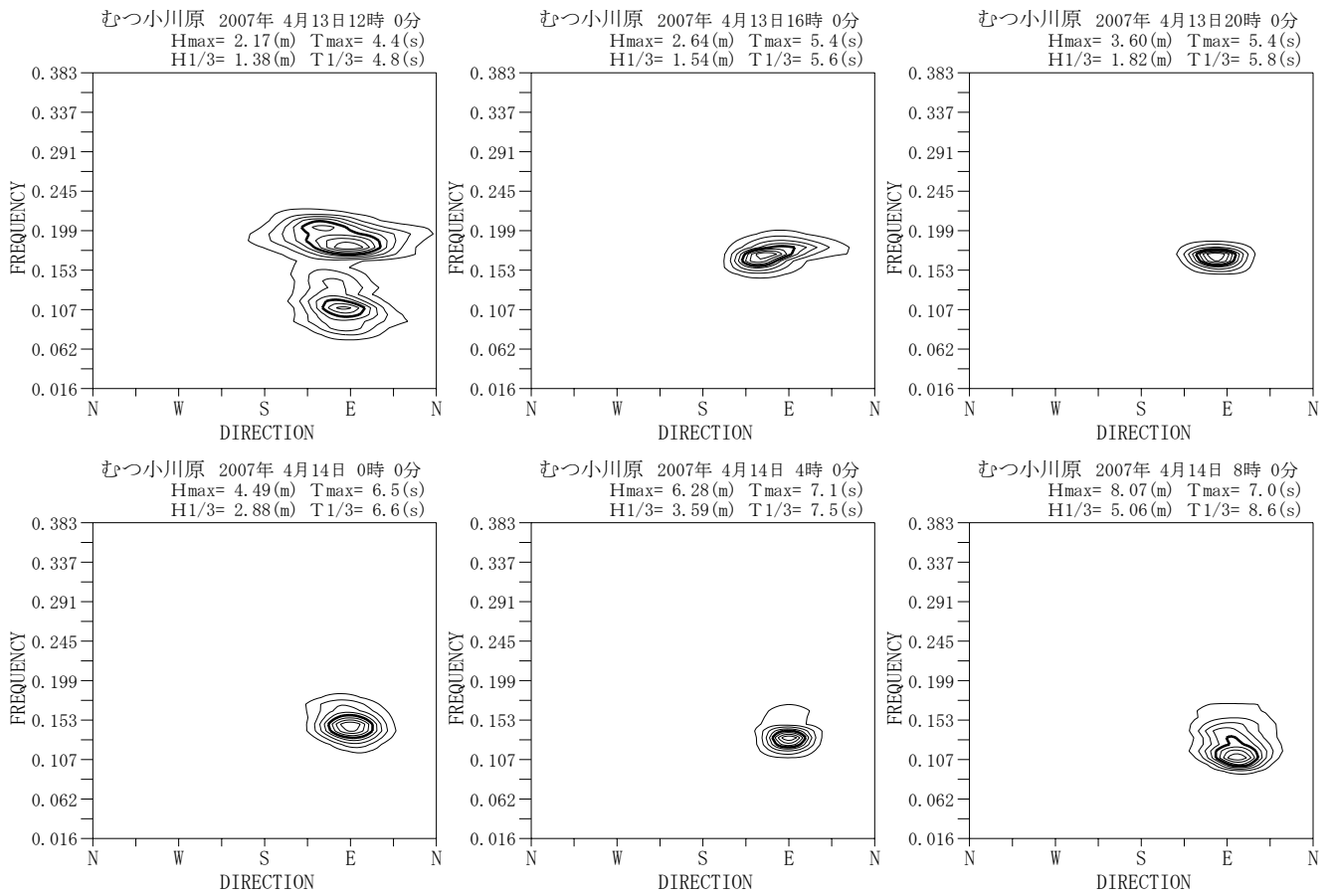
付図-A. 5.31 むつ小川原 代表的な高波期間中の方向スペクトル
