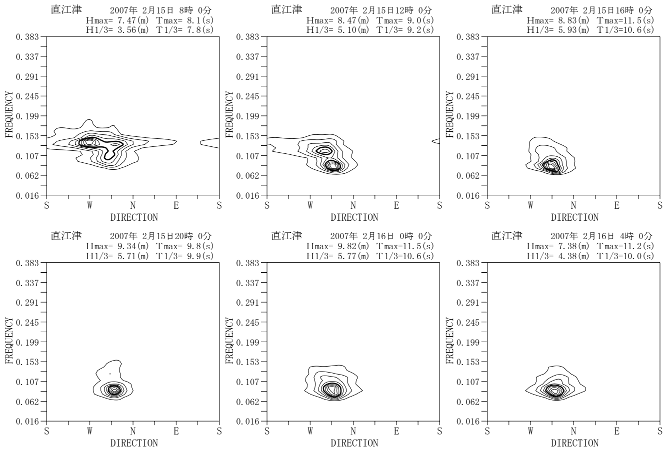
付図-A.5.9 直江津 代表的な高波期間中の方向スペクトル
