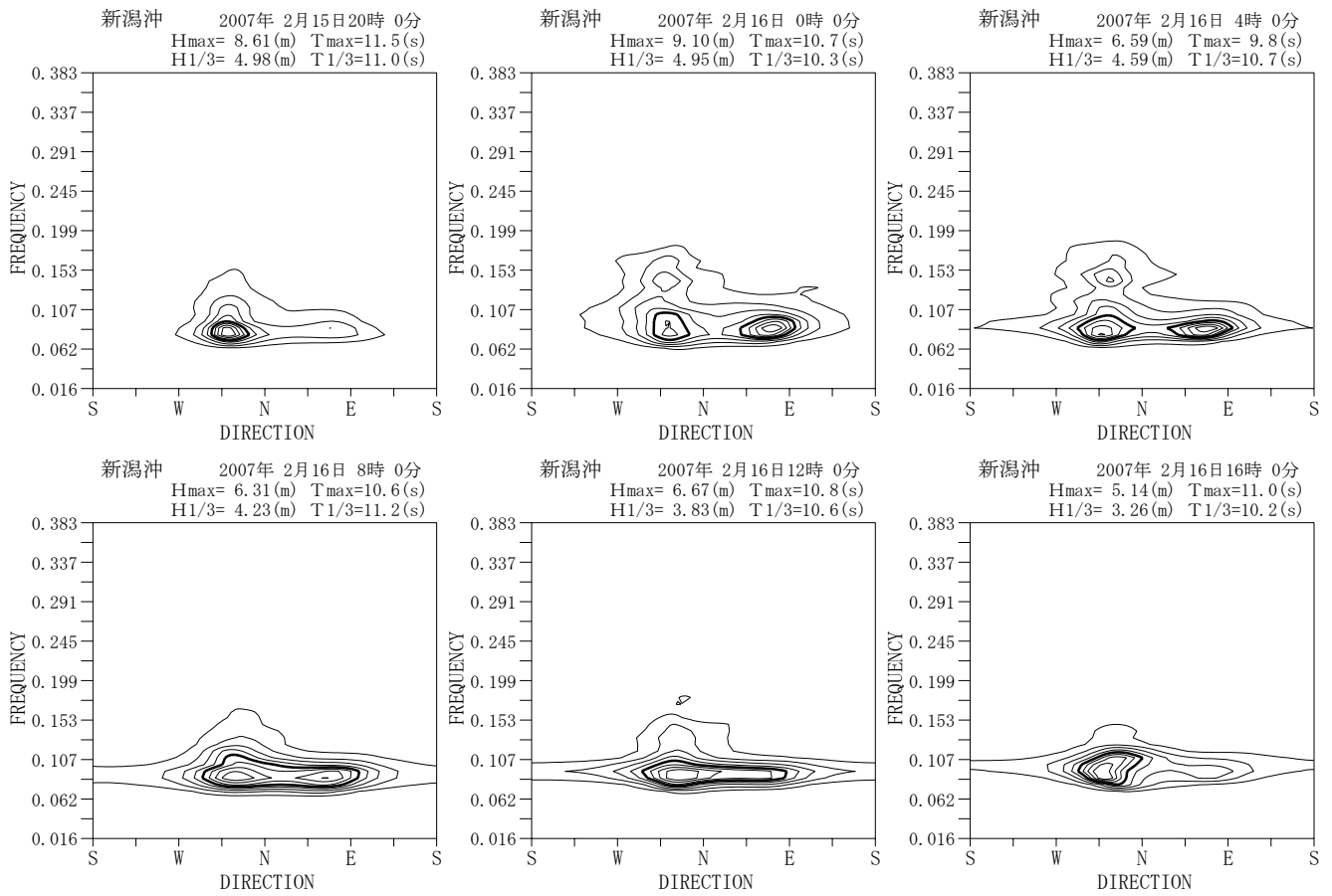
付図-A. 5. 8 新潟沖 代表的な高波期間中の方向スペクトル
