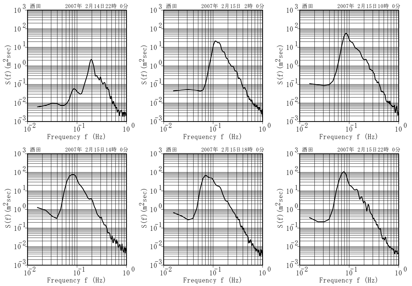
付図-A. 5. 7 酒田 代表的な高波期間中のスペクトル
