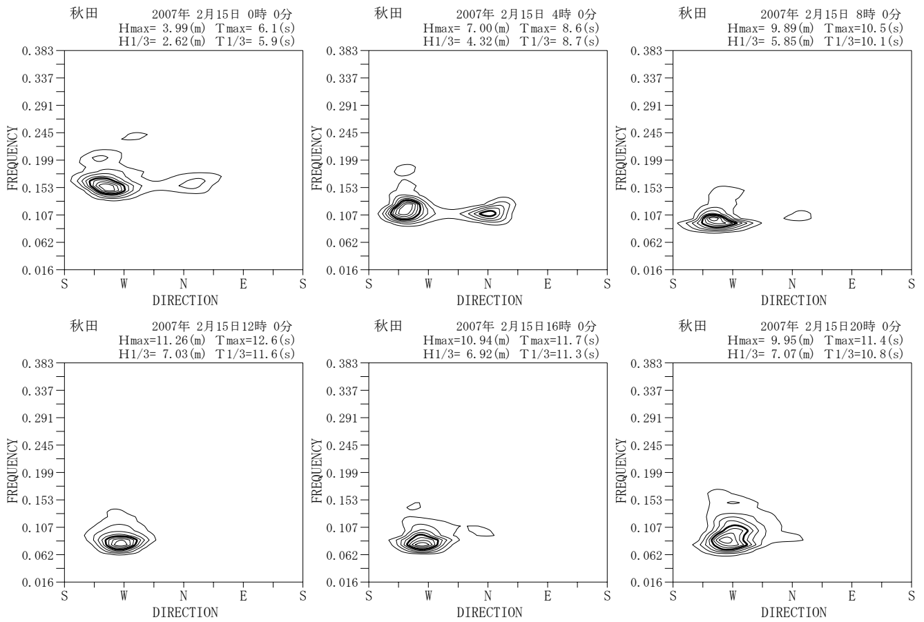
付図-A. 5. 6 秋田 代表的な高波期間中の方向スペクトル
