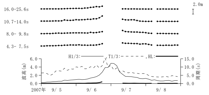
付図-A.3.43 アシカ島 周期帯別波浪特性の経時変化(高波期間中)
