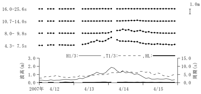
付図-A.3.43 アシカ島 周期帯別波浪特性の経時変化(高波期間中)
