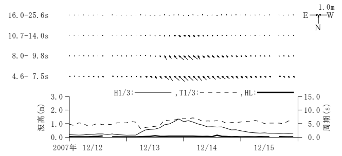
付図-A.3.61 石垣沖 周期帯別波浪特性の経時変化(高波期間中)
