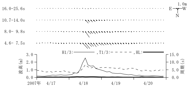
付図-A.3.61 石垣沖 周期帯別波浪特性の経時変化(高波期間中)
