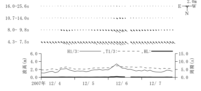
付図-A.3.2 石狩新港 周期帯別波浪特性の経時変化(高波期間中)
