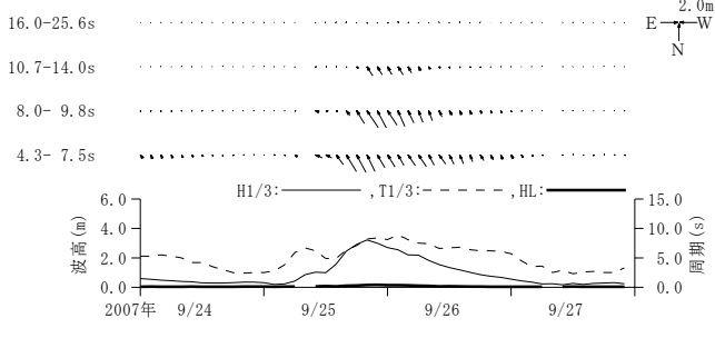
付図-A.3.2 石狩新港 周期帯別波浪特性の経時変化(高波期間中)
