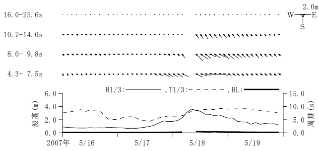
付図-A.3.29 十勝 周期帯別波浪特性の経時変化(高波期間中)
