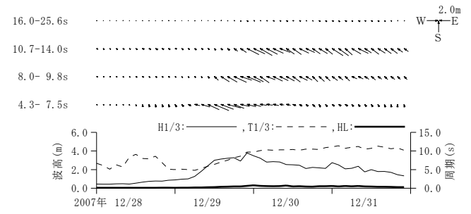
付図-A.3.29 十勝 周期帯別波浪特性の経時変化(高波期間中)
