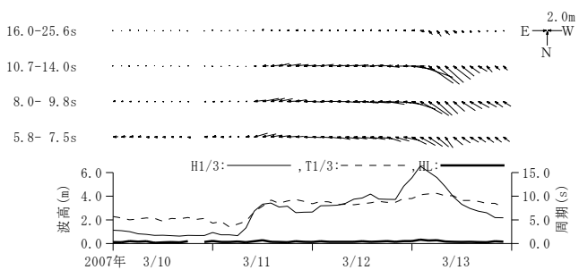
付図-A.3.1 留萌 周期帯別波浪特性の経時変化(高波期間中)
