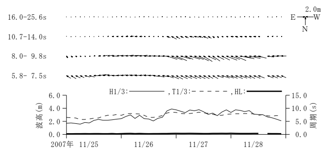
付図-A.3.1 留萌 周期帯別波浪特性の経時変化(高波期間中)
