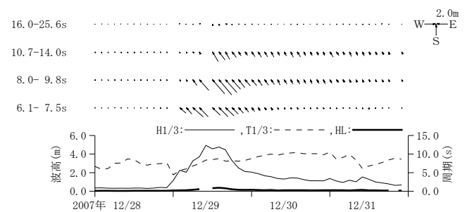
付図-A. 3. 30 苫小牧 周期帯別波浪特性の経時変化(高波期間中)
