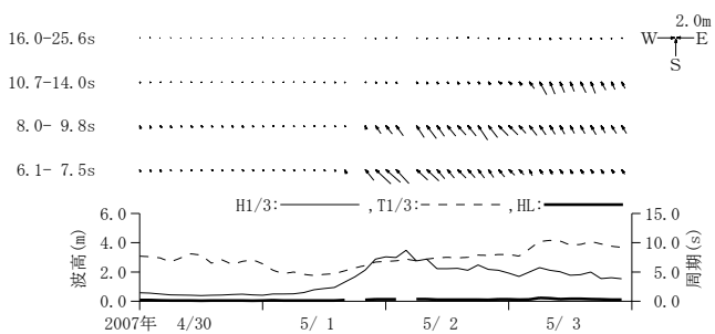
付図-A. 3. 30 苫小牧 周期帯別波浪特性の経時変化(高波期間中)
