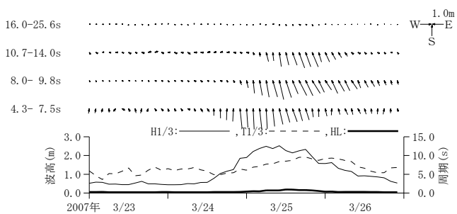
付図-A. 3. 47 御前崎 周期帯別波浪特性の経時変化(高波期間中)
