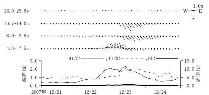
付図-A. 3. 47 御前崎 周期帯別波浪特性の経時変化(高波期間中)
