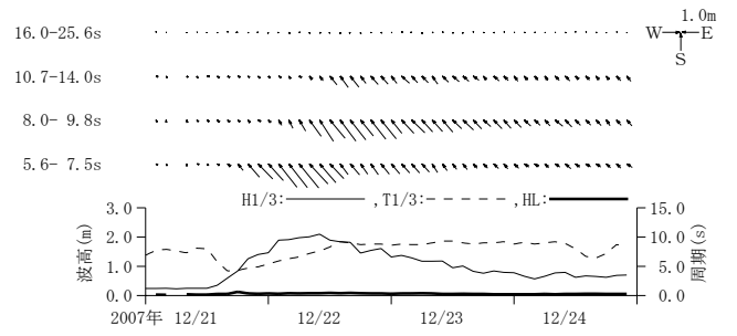
付図-A. 3.57 志布志湾 周期帯別波浪特性の経時変化(高波期間中)
