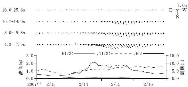
付図-A. 3. 21 藍島 周期帯別波浪特性の経時変化(高波期間中)
