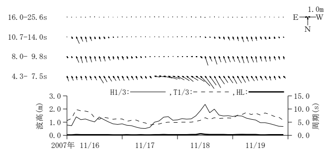
付図-A. 3. 21 藍島 周期帯別波浪特性の経時変化(高波期間中)
