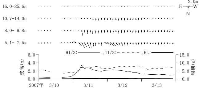
付図-A. 3. 22 玄界灘 周期帯別波浪特性の経時変化(高波期間中)
