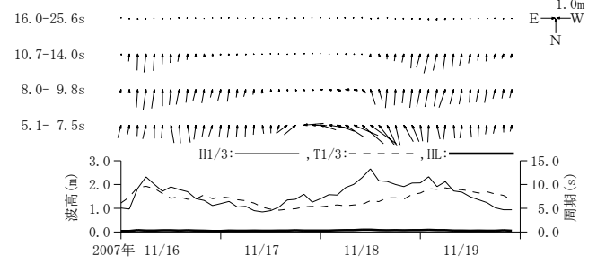
付図-A. 3. 22 玄界灘 周期帯別波浪特性の経時変化(高波期間中)
