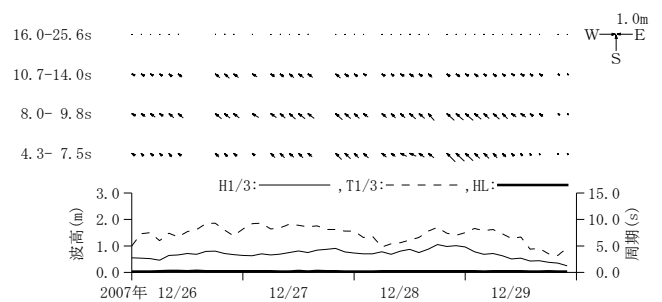
付図-A. 3. 51 小松島 周期帯別波浪特性の経時変化(高波期間中)
