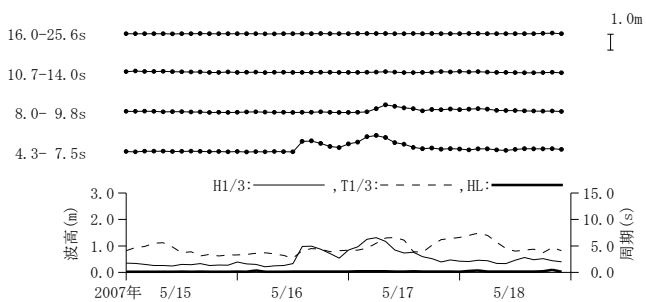
付図-A. 3. 51 小松島 周期帯別波浪特性の経時変化(高波期間中)
