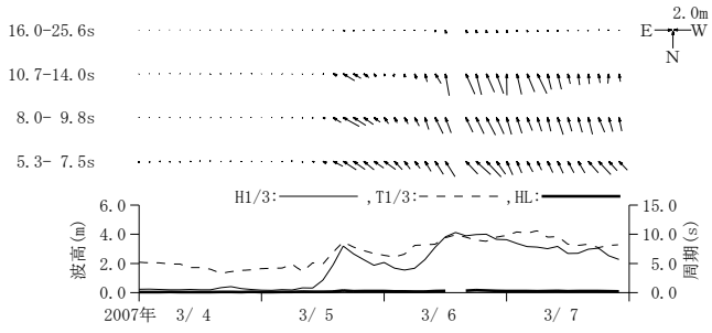
付図-A. 3. 16 柴山 周期帯別波浪特性の経時変化(高波期間中)
