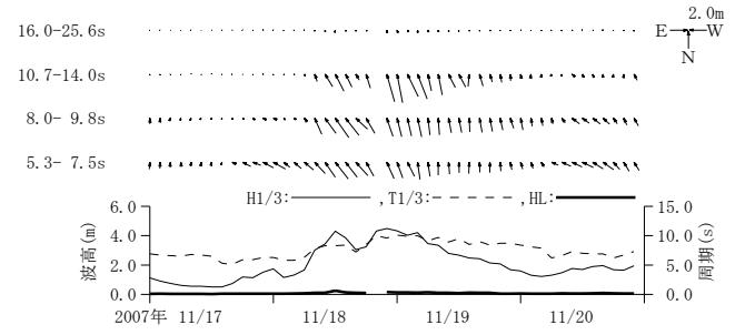
付図-A. 3. 16 柴山 周期帯別波浪特性の経時変化(高波期間中)
