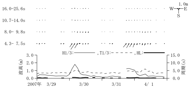
付図-A.3.50 神戸 周期帯別波浪特性の経時変化(高波期間中)
