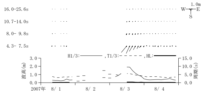
付図-A.3.50 神戸 周期帯別波浪特性の経時変化(高波期間中)
