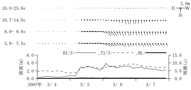
付図-A. 3. 20 浜田 周期帯別波浪特性の経時変化(高波期間中)
