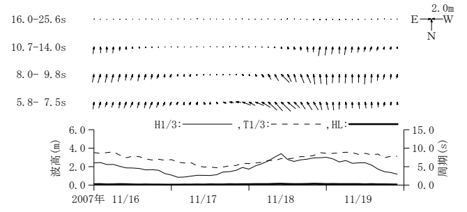
付図-A. 3. 20 浜田 周期帯別波浪特性の経時変化(高波期間中)
