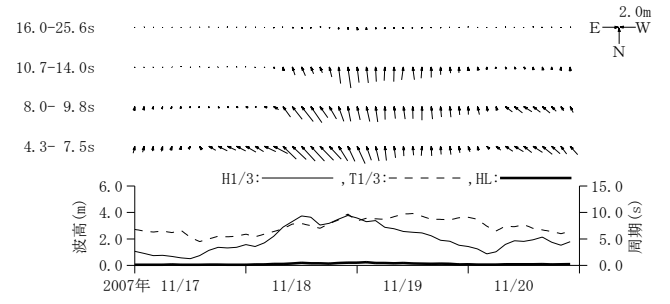
付図-A. 3. 18 鳥取 周期帯別波浪特性の経時変化(高波期間中)
