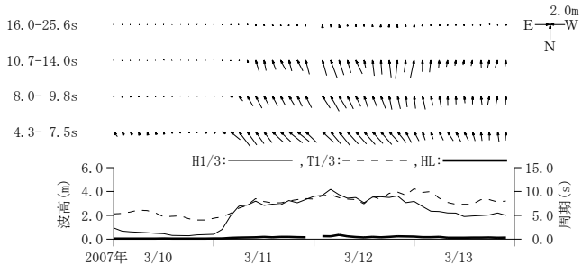
付図-A. 3. 18 鳥取 周期帯別波浪特性の経時変化(高波期間中)
