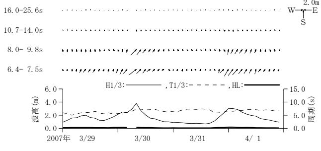
付図-A. 3. 49 潮岬 周期帯別波浪特性の経時変化(高波期間中)
