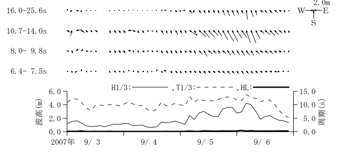
付図-A. 3. 49 潮岬 周期帯別波浪特性の経時変化(高波期間中)
