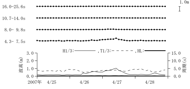
付図-A.3.4 青森 周期帯別波浪特性の経時変化(高波期間中)
