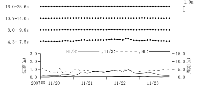
付図-A.3.4 青森 周期帯別波浪特性の経時変化(高波期間中)
