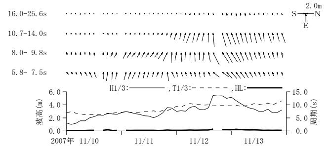
付図-A. 3. 33 久慈 周期帯別波浪特性の経時変化(高波期間中)
