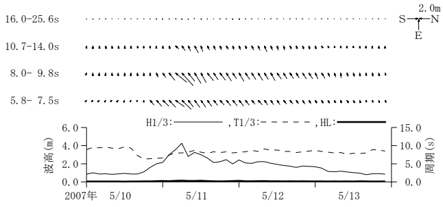
付図-A. 3. 33 久慈 周期帯別波浪特性の経時変化(高波期間中)
